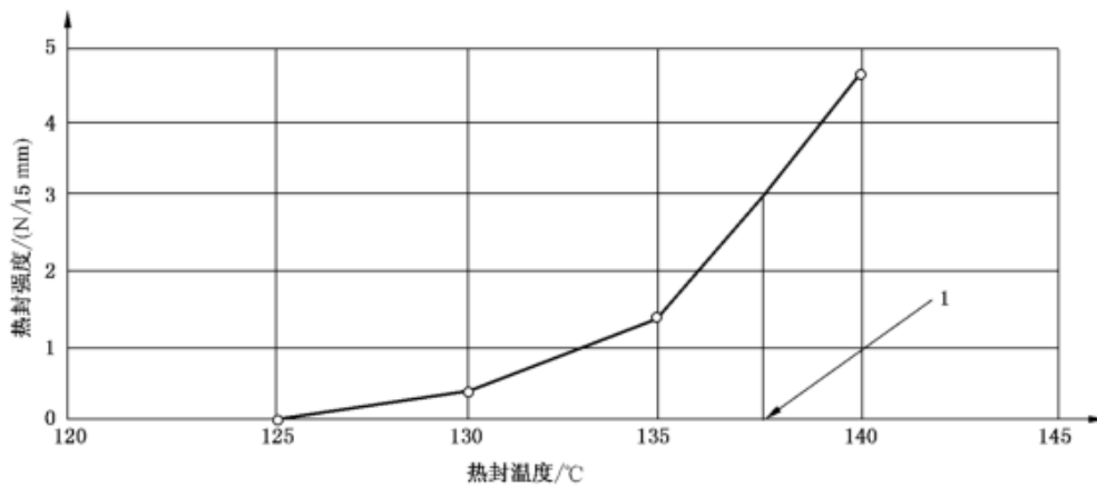
图 1 起始热封温度的判定
